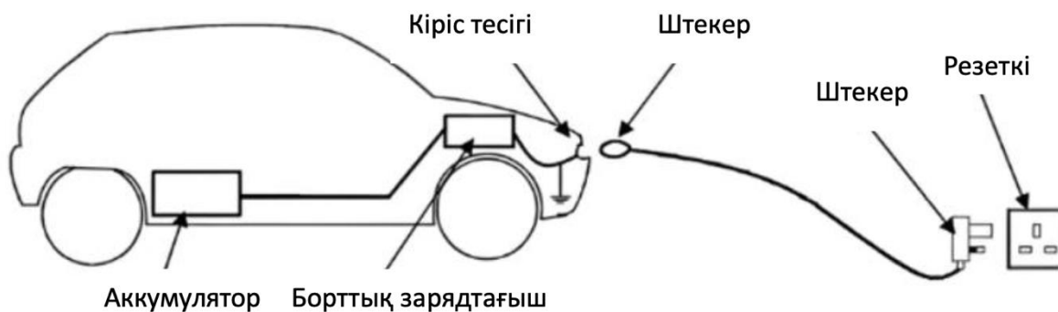
1-сурет. Электромобильді 1-деңгейде зарядтау
