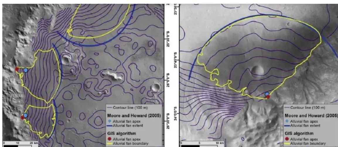
Рис. 6 Картографирование конуса выноса на Марсе посредством ГИС-алгоритма. [5]
