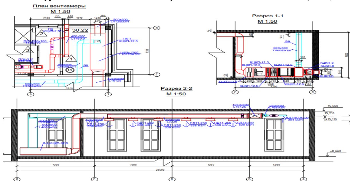
Рис.1 Подбор и компоновка оборудования кондиционирования
