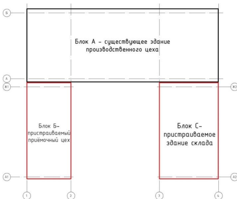
Рисунок 1 Блокировка здания завода с существующим производственным цехом и пристроиваемыми зданиями складирования и приема.
