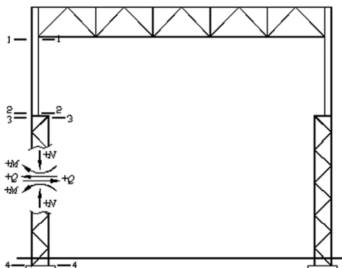
Рис. 1. Нумерация сечений стойки поперечной рамы
