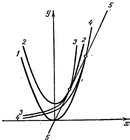
Рис. 5. 1 — кривая y = x^2 ; 2 — кривая y = x^2 + 1 ; 3 — кривая y = (2/e)^2 e^x ; 4 — кривая y = (2/e)^2 e^x ; 5 — прямая y = 2x .
